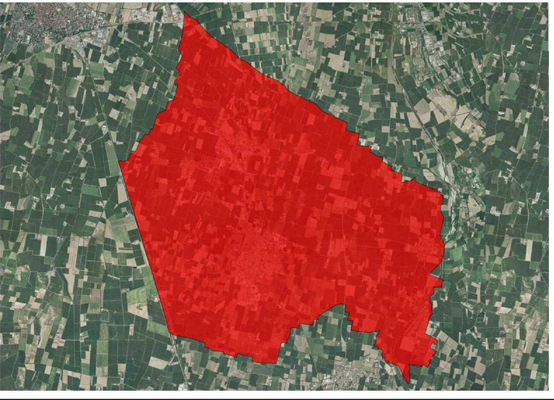
Tav. 03: CARTA IDROGEOLOGICA E DELLA VULNERABILITÀ DELLA FALDA DEL TERRITORIO COMUNALE (SCALA 1:10.000)
